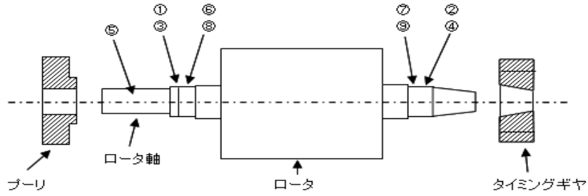
2-1 ロータ軸ベアリング嵌合部測定記録(単位:1/100mm)
