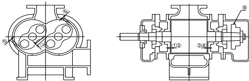
2-3 クリアランス測定値
